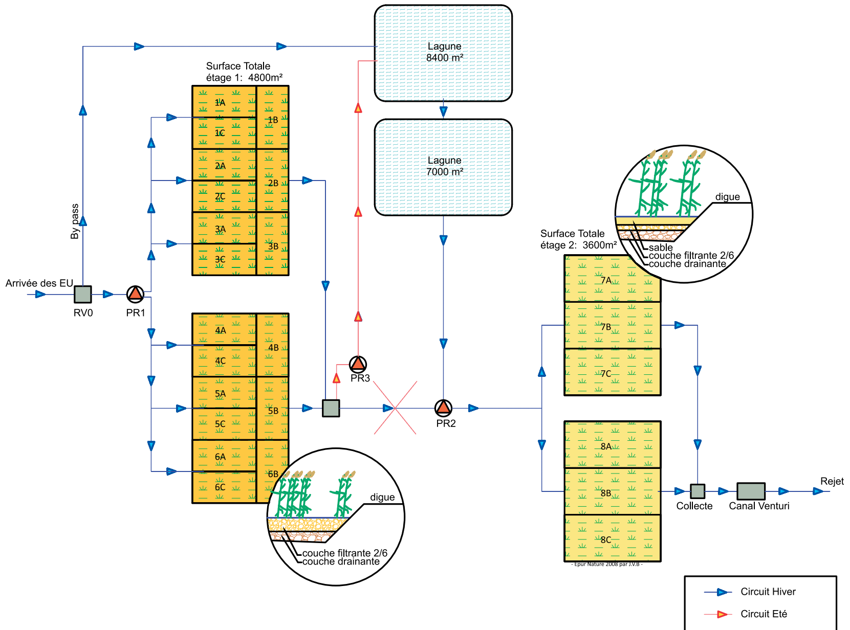
- schéma de la station d'épuration de NEGREPELISSE - 4000EH -
